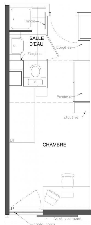
CHAMBRE INTERNAT
